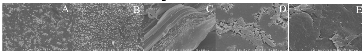
تصویر ۳: تصاویر sem نانو ذرات نقره در غلظت‌های مختلف دارای رنج ۲۰-۳۰ نانومتر نشان می‌دهد (فرنس شماره ۹)
