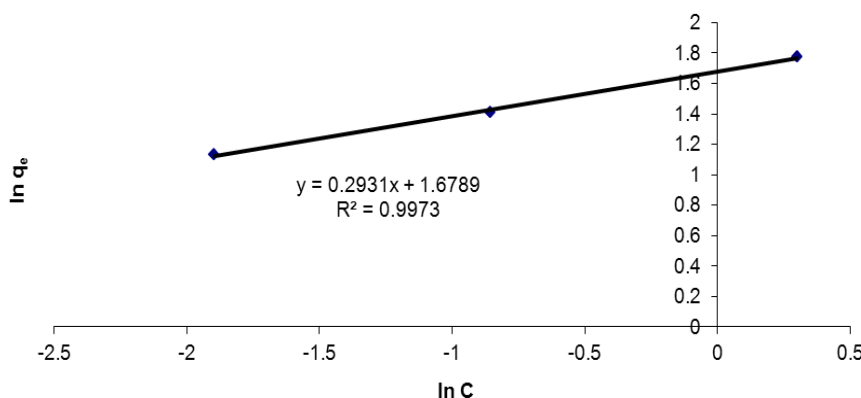
نمودار ۴. ایزوترم فروندلیج جذب رنگ بر نانوتیوب کربنی تک جداره
